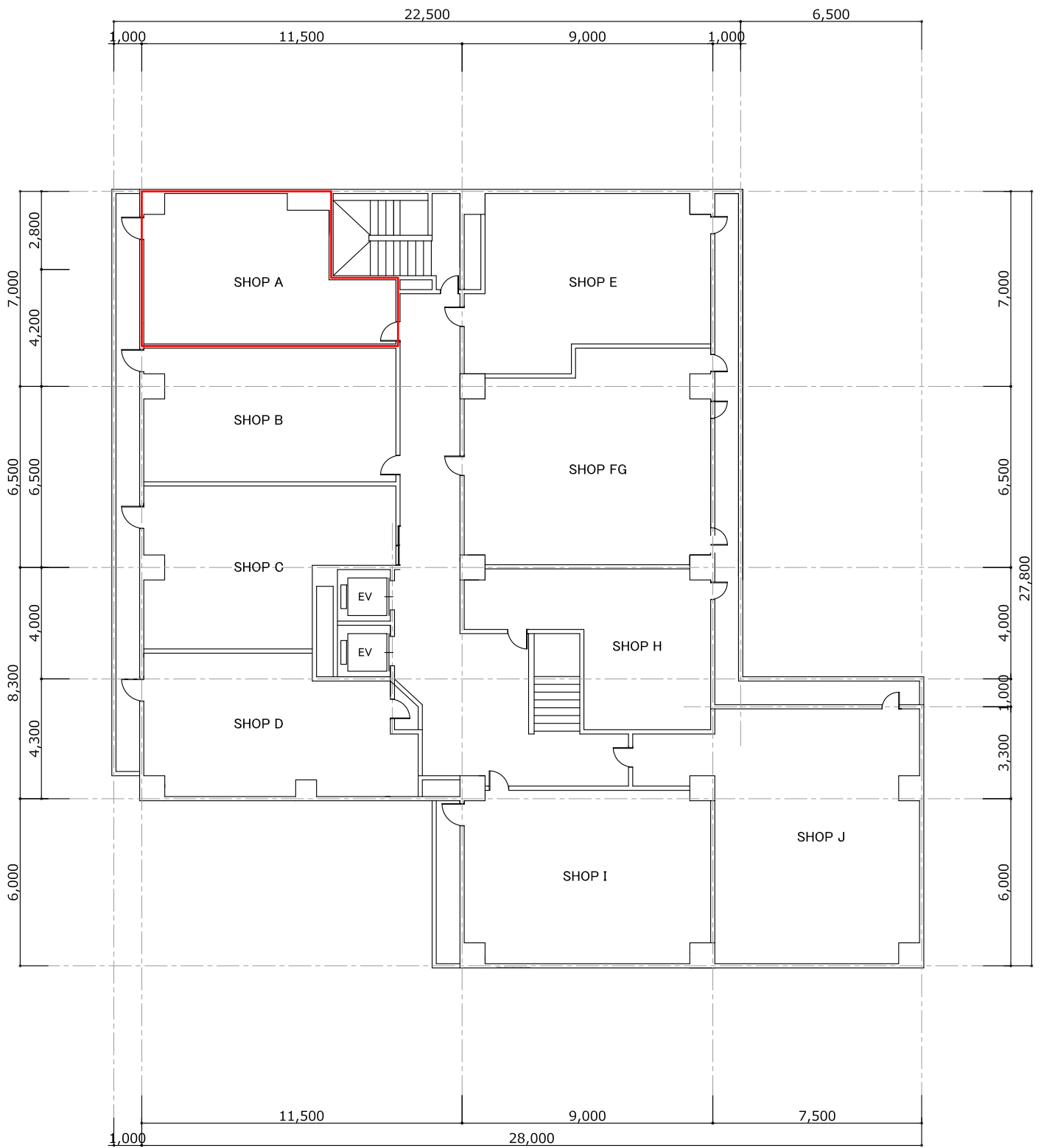
横浜エクセレントⅢ 地下1階平面図
